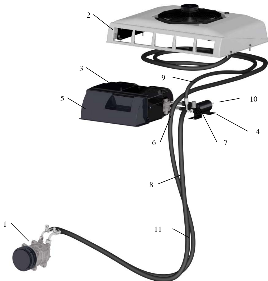
Рис. 2. Состав системы кондиционирования:
