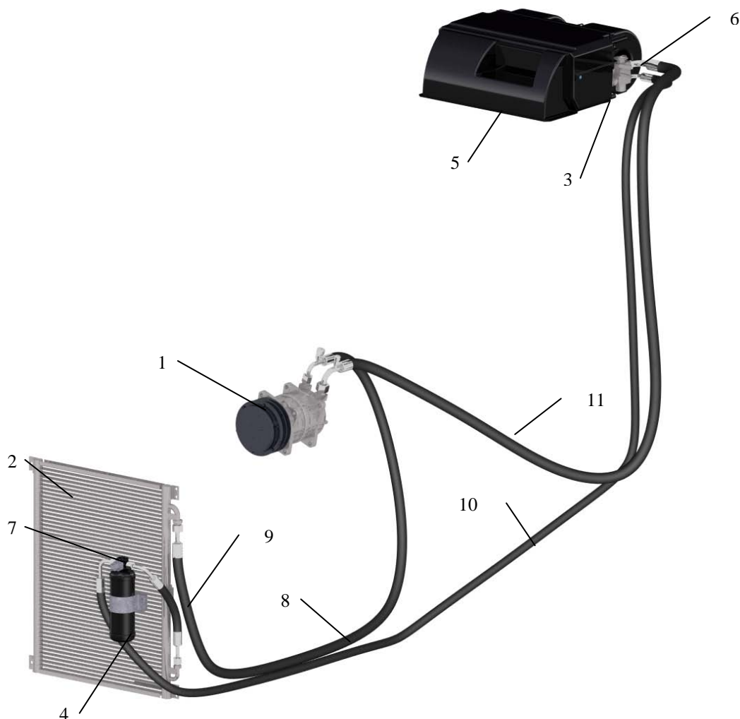
Рис. 1. Состав системы кондиционирования:
